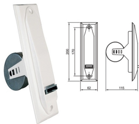
RECOGEDOR PERSIANA EMBUTIR PLASTICO 22MM BLAN
